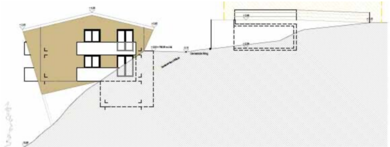
ANSICHT OST 1:100
