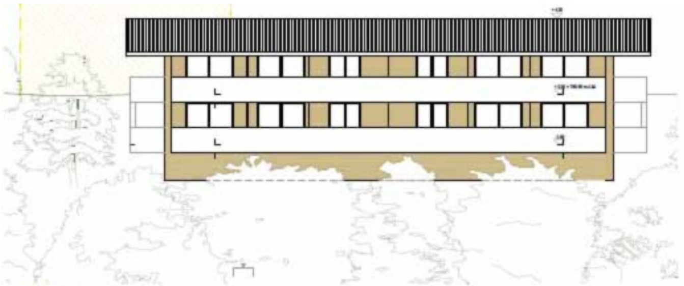
ANSICHT SÜD 1:100
