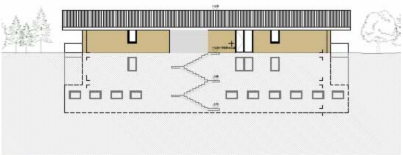
ANSICHT NORD 1:100
