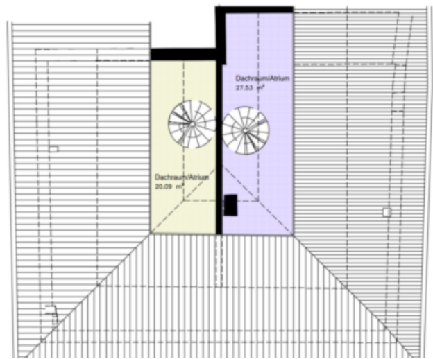
GRUNDRISS DACHGESCHOSS 1:100
