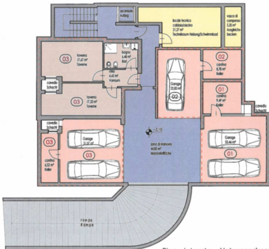
Piano interrato - Untergeschoss
