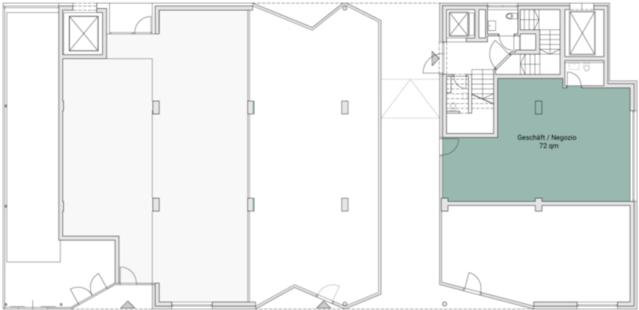
ERDGESCHOSS
