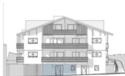
Südansicht Prospetto sud
