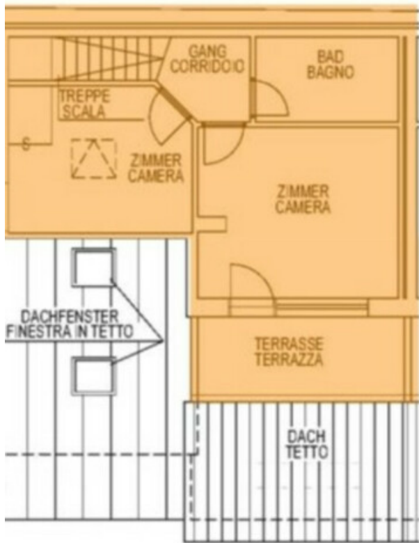
TTES OBERGESCHOSS TERZO PIANO
