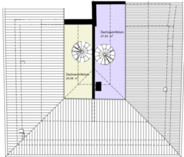
GRUNDRISS DACHGESCHOSS 1:100
