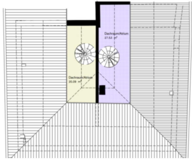
GRUNDRISS DACHGESCHOSS 1:100
