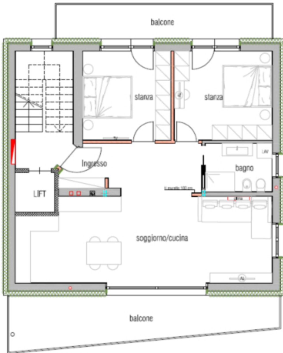
PLANIMETRIA PIANO SECONDO - SCALA 1:100 SOL.2
