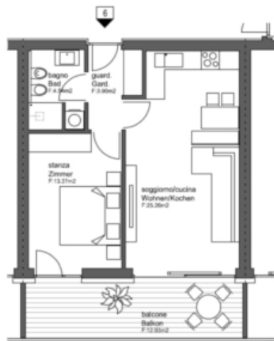
WOHNUNG 6 - APPARTAMENTO 6
