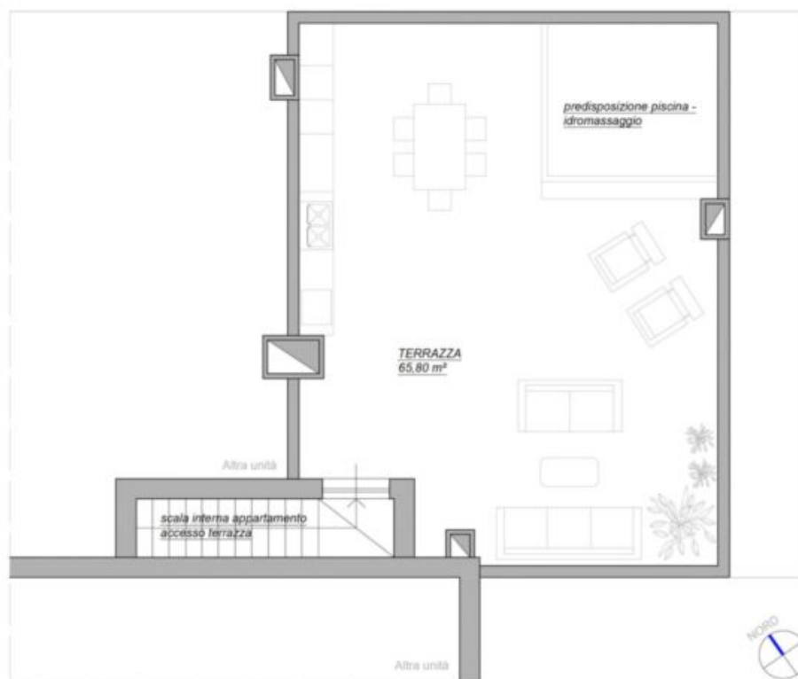
PLANIMETRIA TERRAZZA | 3° PIANO | ATTICO STATO DI PROGETTO
