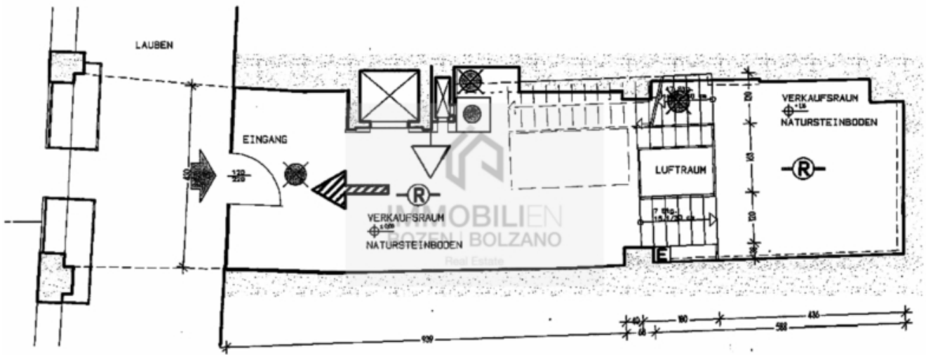
ERDGESCHOSS 1:100
