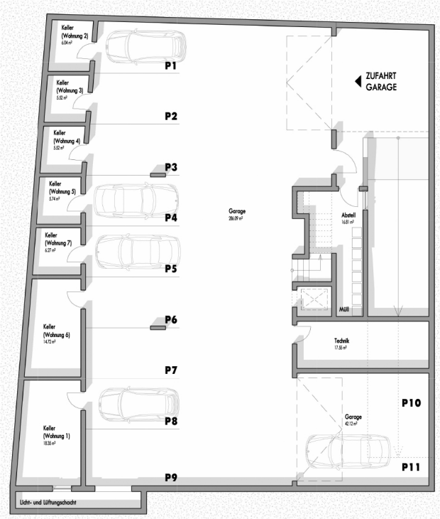
KELLERGESCHOSS
