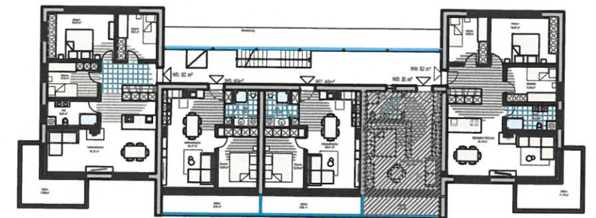
OBERGESCHOSS
