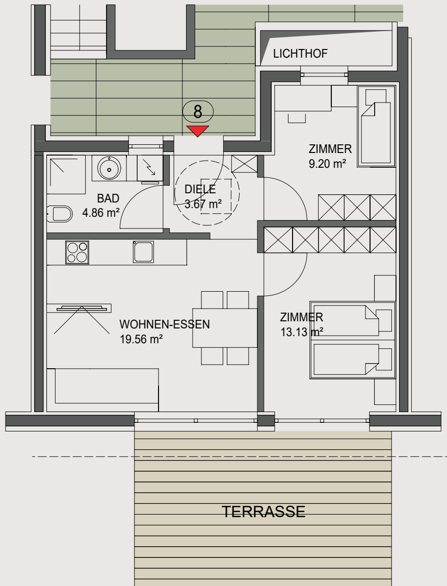
WOHNEINHEIT 8 50,39 m²
