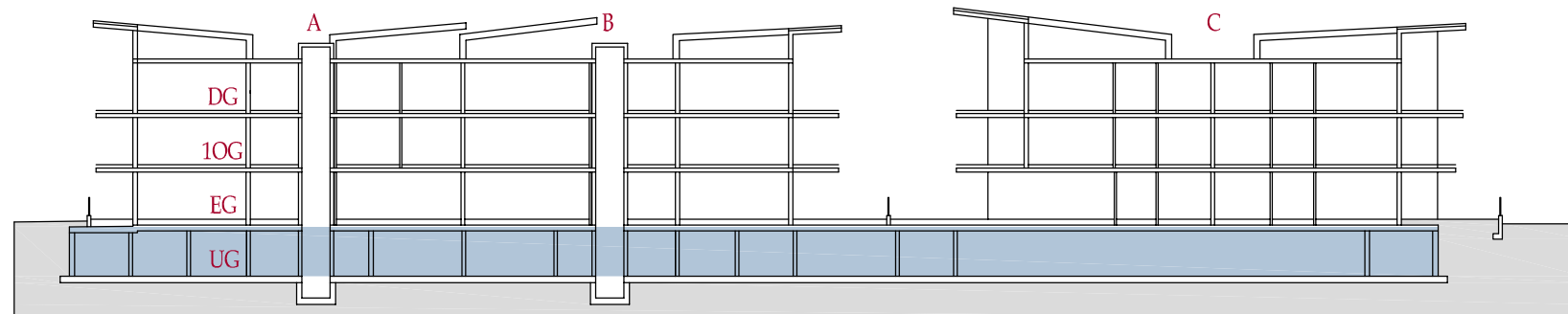
Schnitt - sezione
